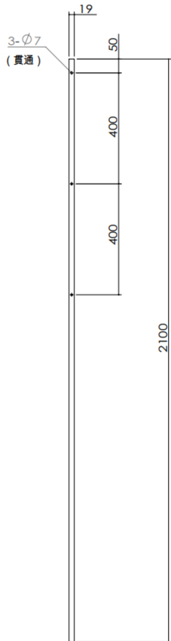
パネル用アーム加工 詳細図 ( S = 1 : 10 )
