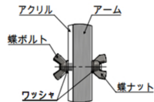
詳細図 A (S = 1 : 2.5)
