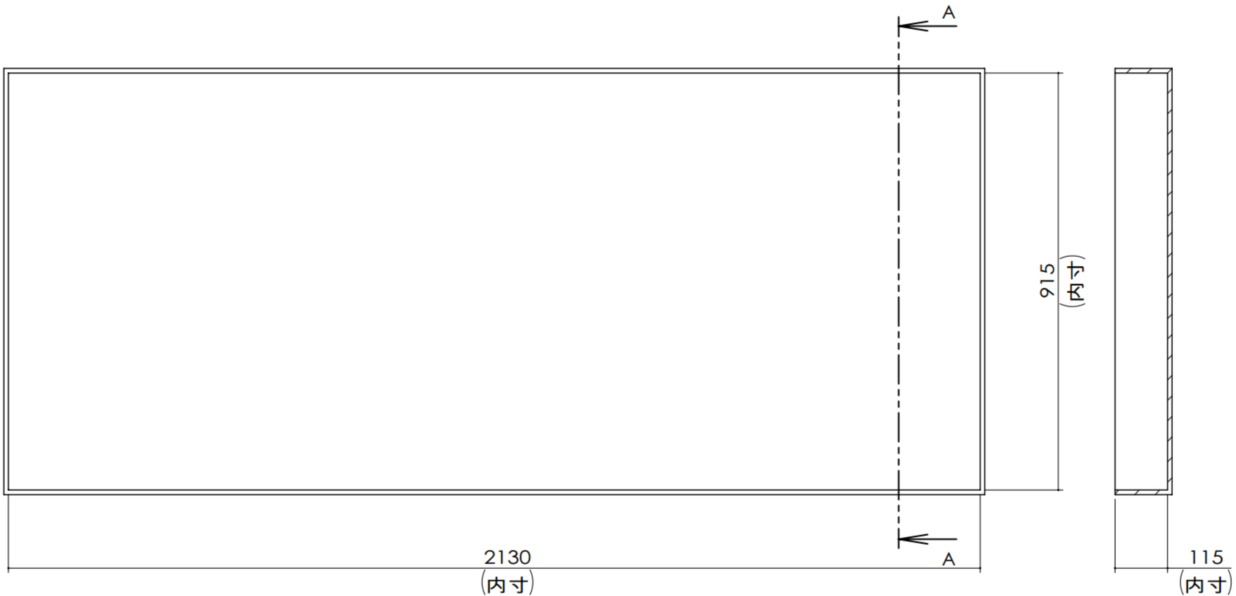
断面図 A-A
