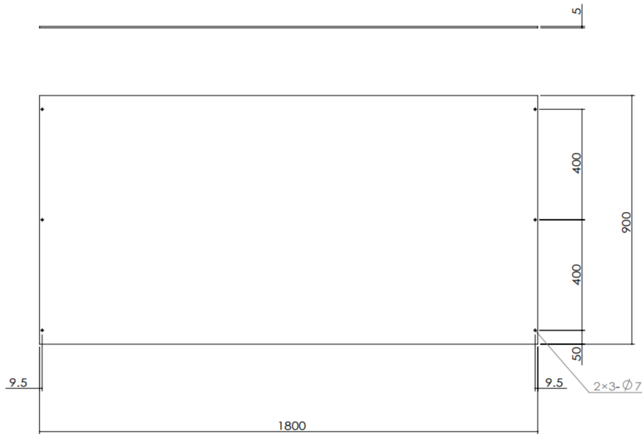
透明アクリルパネル 詳細図 ( S = 1 : 10 )
