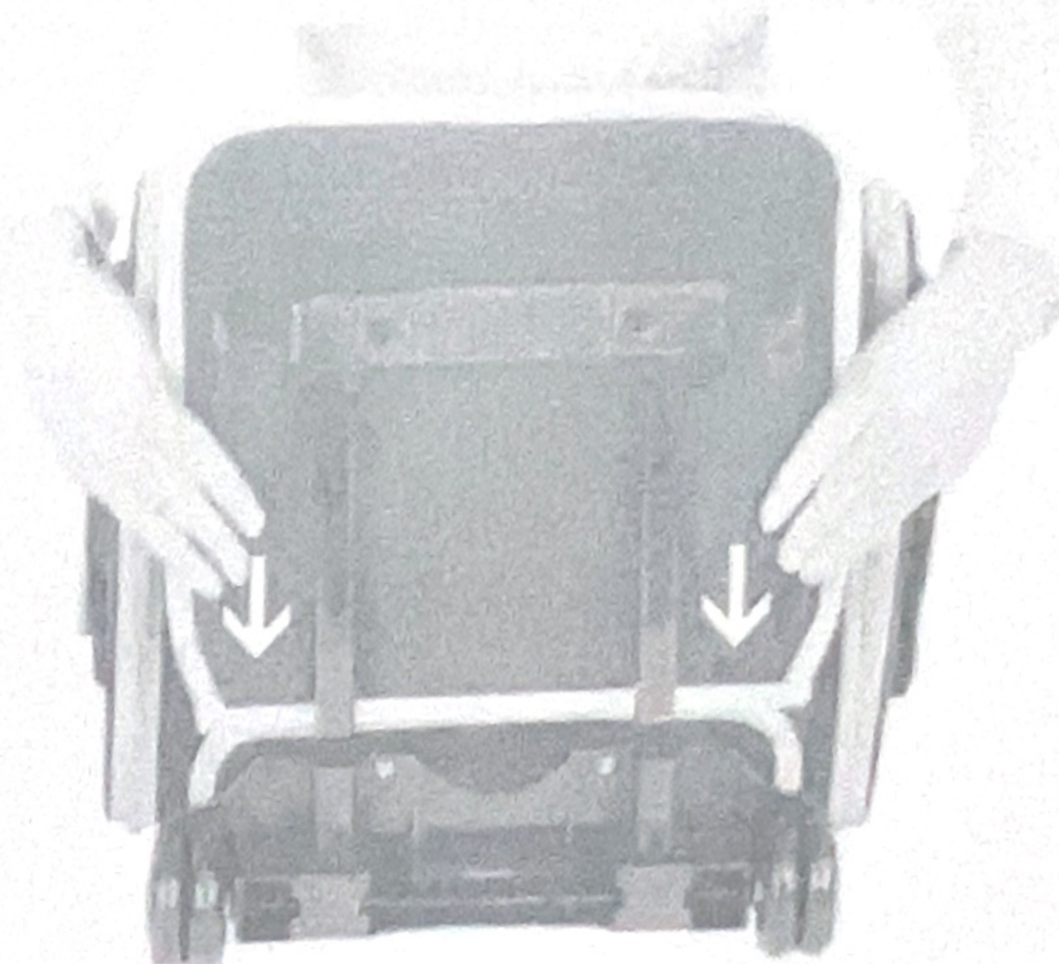
②ステップ2 底部の補助バーを本体に差し込める
